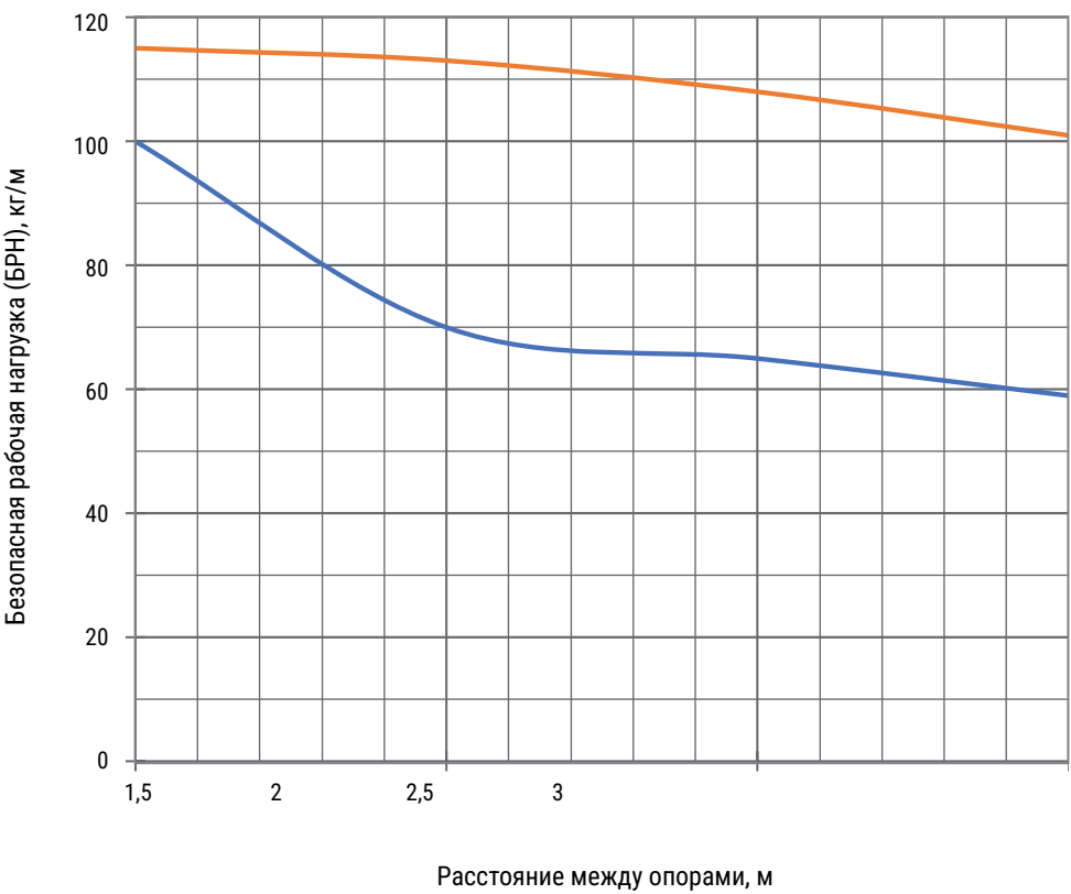
График нагрузок
