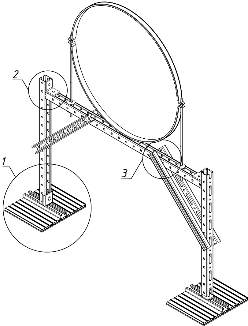
Схема опор Н7.2.1-9
